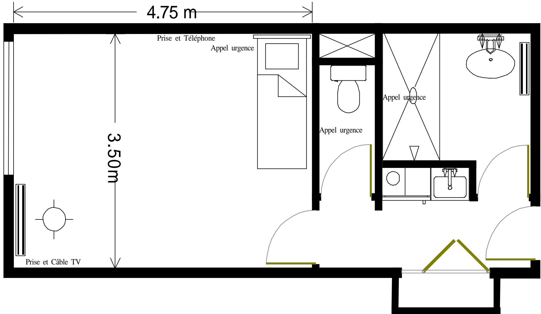
Plan d'un studio
